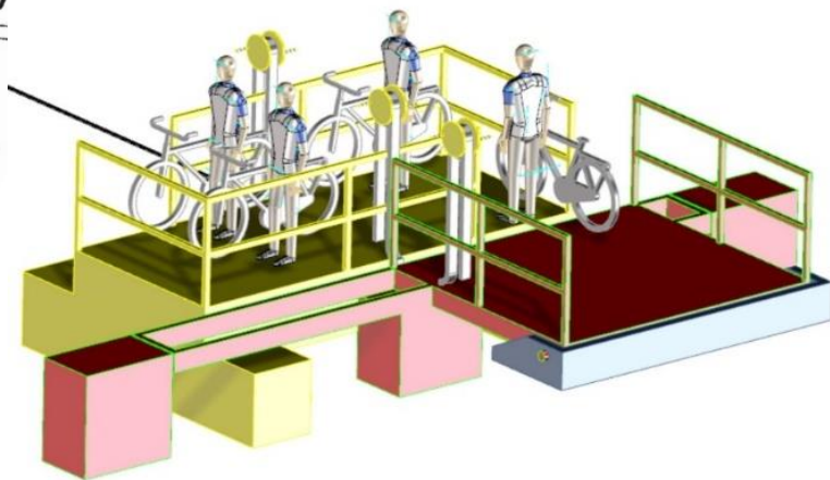
Situatietekening fietspont
