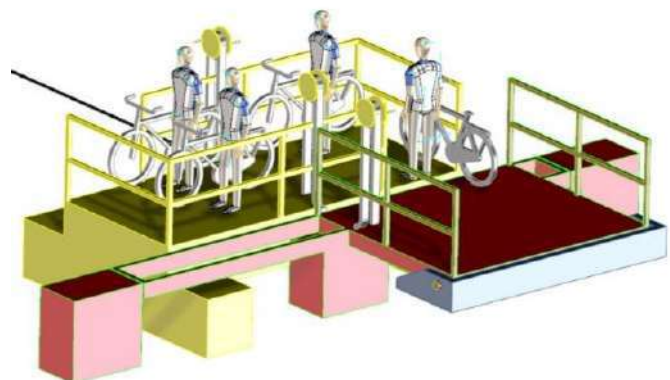
Situatietekening fietspont
